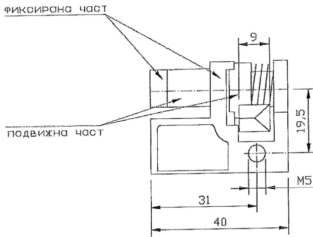
Фигура 1 - Галванизиран стоманен ключ и халф цилиндър тип „Полумесец“
